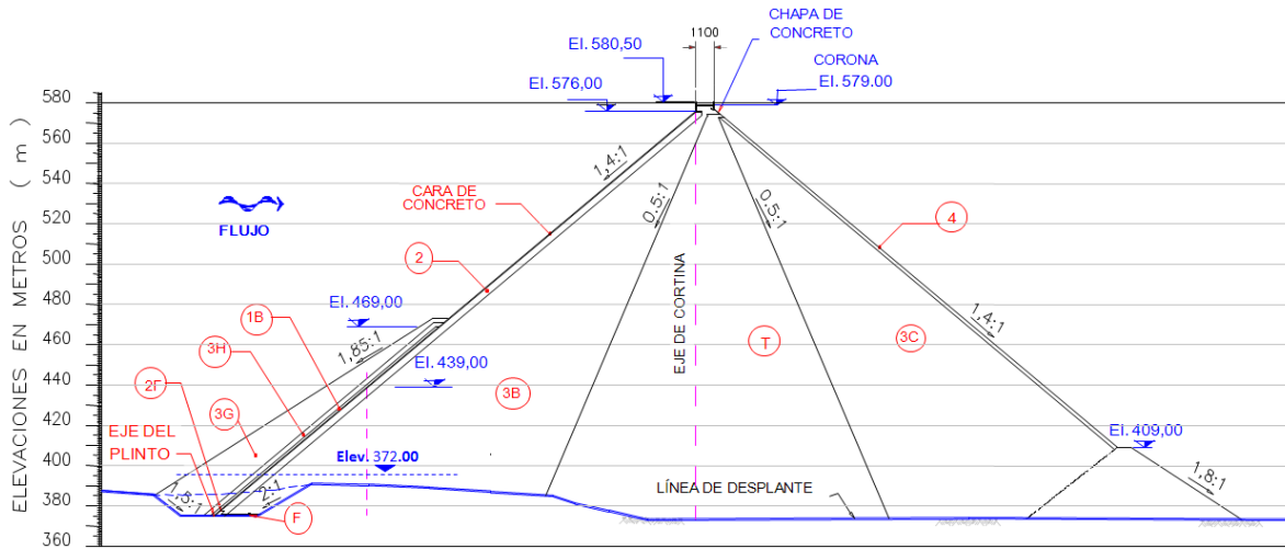
SECCIÓN TRANSVERSAL DE LA CORTINA
