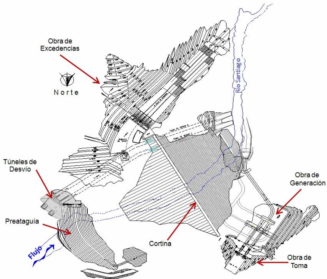
ARREGLO GENERAL DE LAS OBRAS PRINCIPALES
